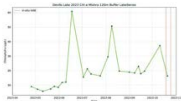
Chlorophyll-a values in Devils Lake, 2023.
